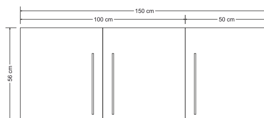
HS 150 - Skizze
